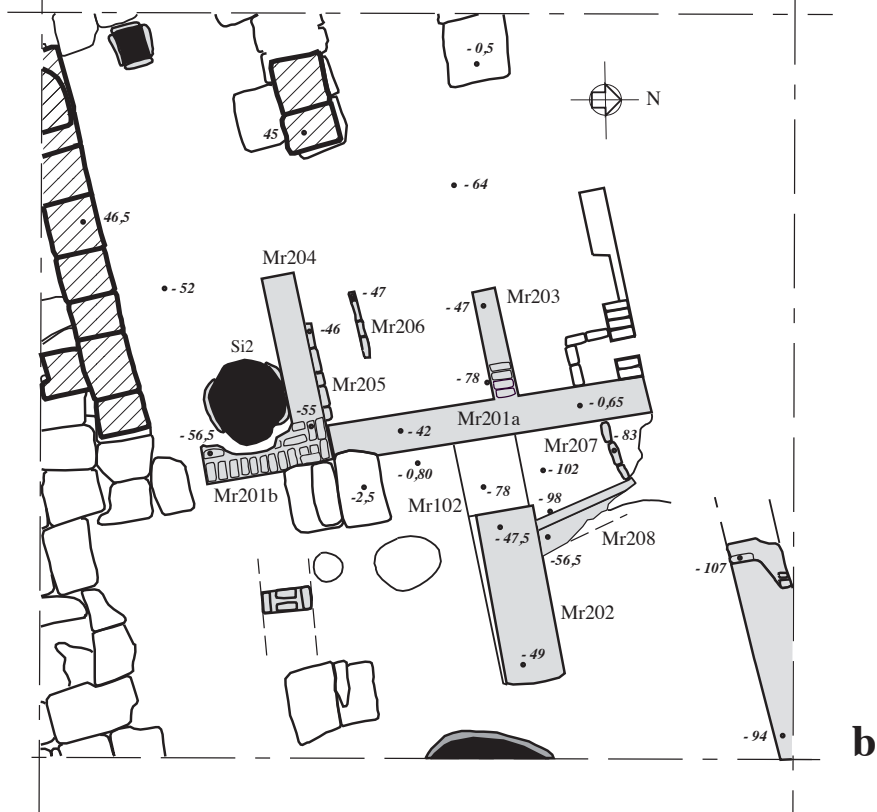
Fig. 1, a et b (Dessin : Michel AZIM) : les deux états successifs des substructures de brique à l'angle nord-est des ruines du temple A ; les altitudes sont données à partir du point zéro du temple, à 160,69 m.
