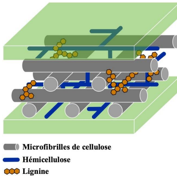
Fig. 1 : Schéma simplifié de la composition de la paroi cellulaire des végétaux représentant l'entrelacement de la cellulose, de la lignine et de l'hémicellulose.
