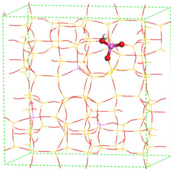
HZSM-5
