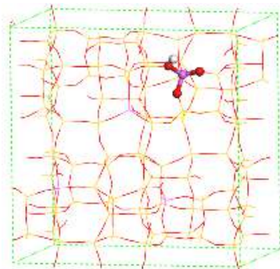
HZSM-5
