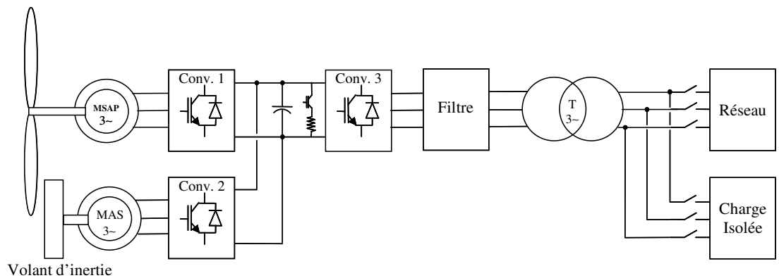
Figure 8. Eolienne à vitesse variable associée à du stockage en vue d'un fonctionnement sur réseau ou sur charges isolées
