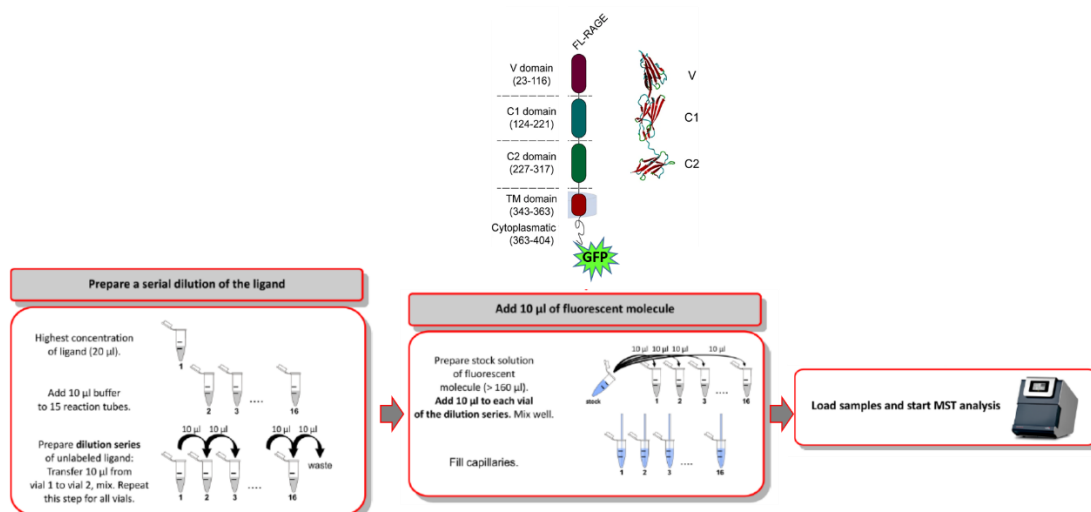
Figure 26 : Protocole simplifié d'une expérience de thermophorèse à microéchelle
