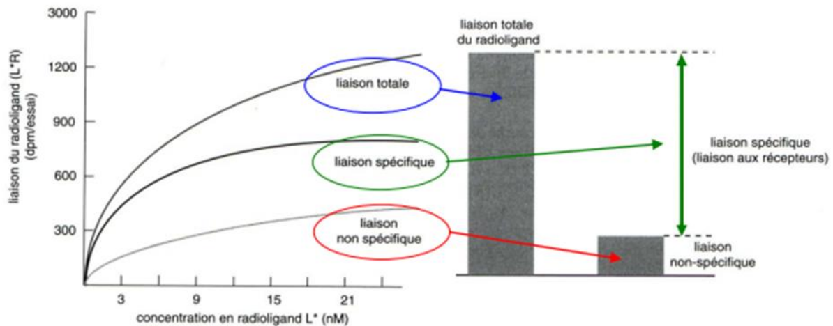
Figure 18 : Expérience de saturation. Détermination du K_d spécifique à l'équilibre.
