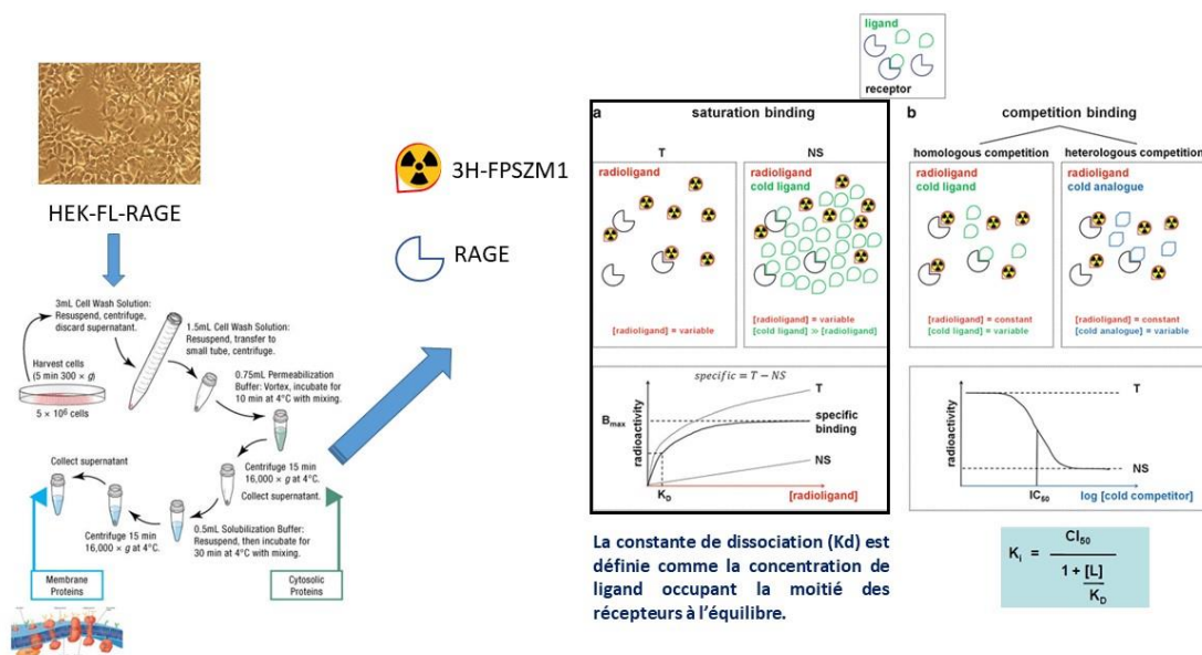
Figure 16 : Principe de la méthode d'étude de l'affinité et de la fonctionnalité de ligands potentiels de RAGE à l'aide d'un radioligand.
