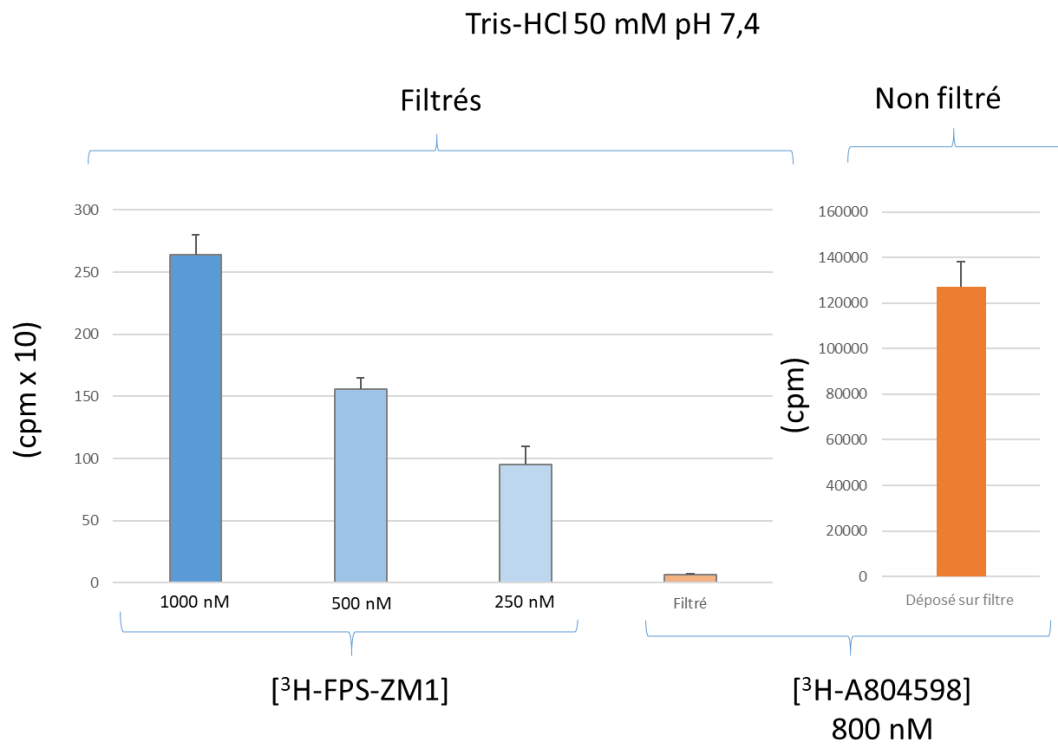
Figure 21 : Etude de l'interaction ligand – filtre ( 3 H-FPS-ZM1 versus 3 H-A804598 (ligand de référence du récepteur P2X7).
