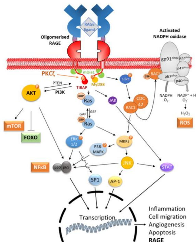
Figure 10 : Signalisation intracellulaire de RAGE. L'oligomérisation de RAGE lors de la liaison du ligand provoque sa phosphorylation sur la Ser391 par la PKC \zeta , recrutant ainsi TIRAP et MyD88, et induisant l'activation de mDIA1. La voie PI3K/AKT/mTOR est activée tandis que FOXO est inhibée. Plusieurs voies MAPK sont également stimulées, activant les voies ERK 1/2, p38-MAPK et JNK. La voie JAK/STAT est également activée. Enfin, la protéine kinase c-Src est également phosphorylée, ce qui active le complexe RAC1/CDC42, puis les MAPK kinases (MKK) et la NADPH oxydase (production de NADP + et d'espèces réactives de l'oxygène). D'importants facteurs de transcription sont impliqués, notamment NF- \kappa B, SP1, AP-1 et les STAT, favorisant l'inflammation, la migration cellulaire, l'angiogenèse, l'apoptose et l'expression de RAGE 36 .
