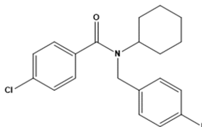
Figure 17 : Précurseur iodé du FPS-ZM1
